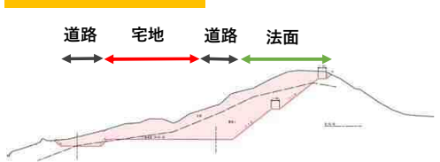
掘削工事（断面図）
