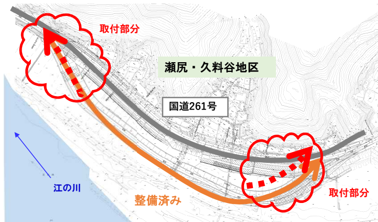
【計画図】
