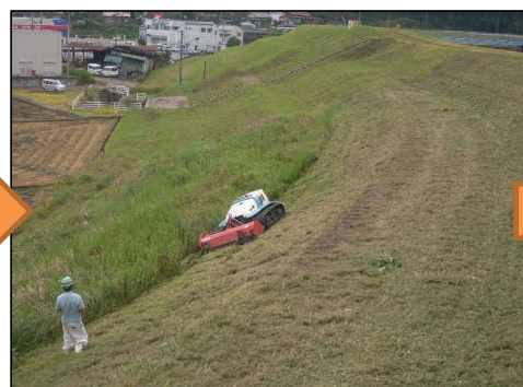
遠隔刈草機による除草
