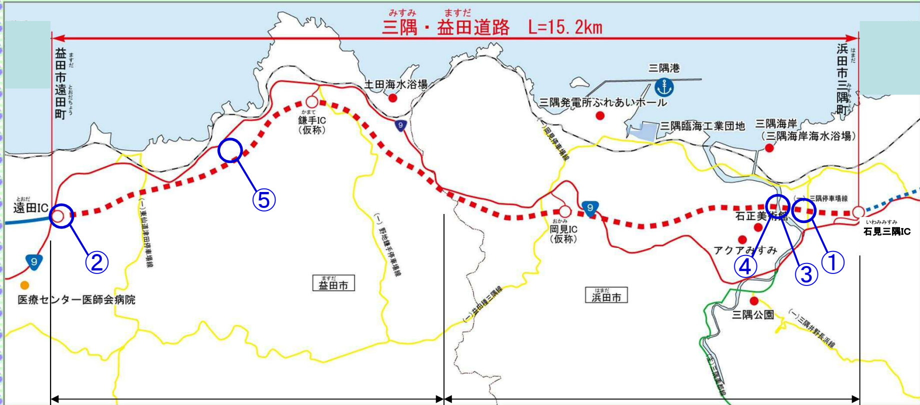
工事位置図
