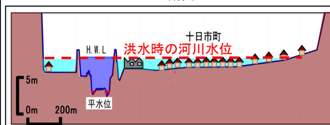
B-B' 断面
