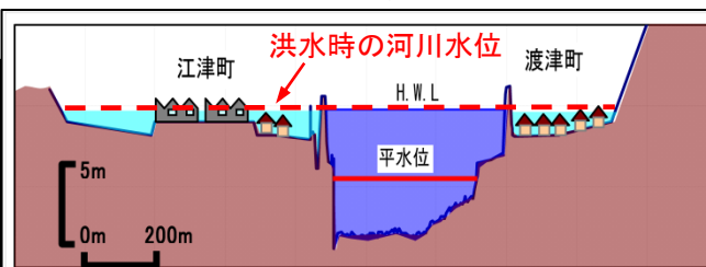
A-A' 断面
