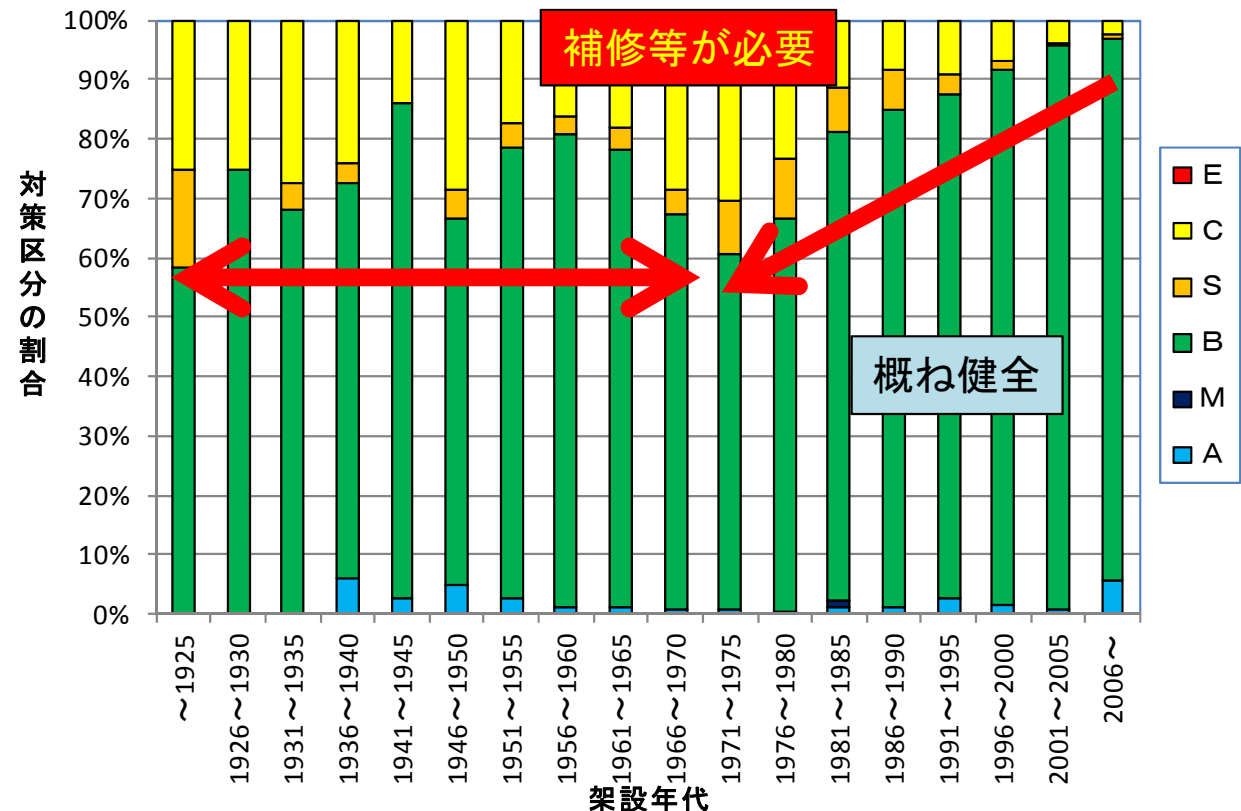
架設年代別対策区分の比率
