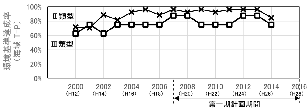
(3) T-P(海域)
