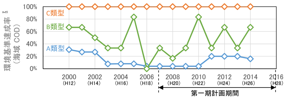
(1) COD(海域)
