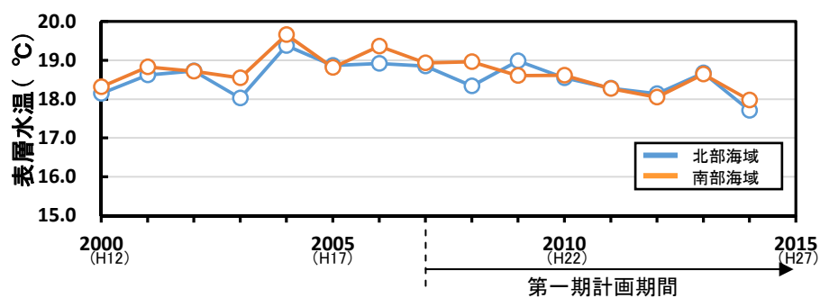
(1) 表層水温
