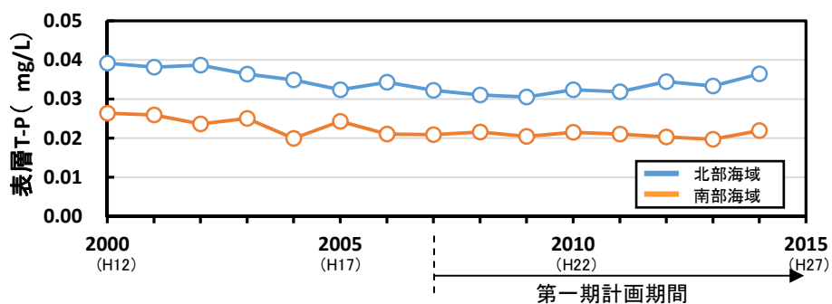
(4) 表層 T-P
