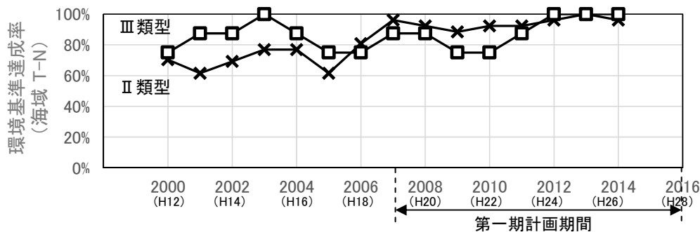
(2) T-N(海域)
