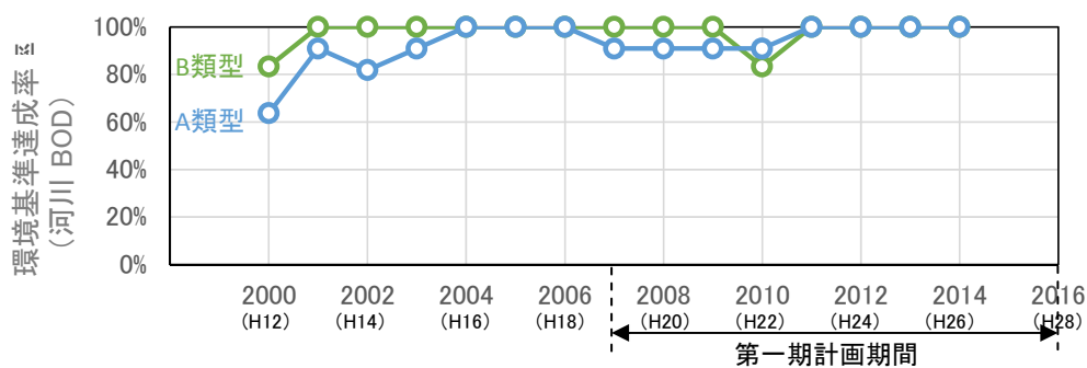
(4) BOD(河川)
