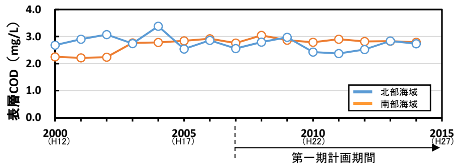
(2) 表層 COD
