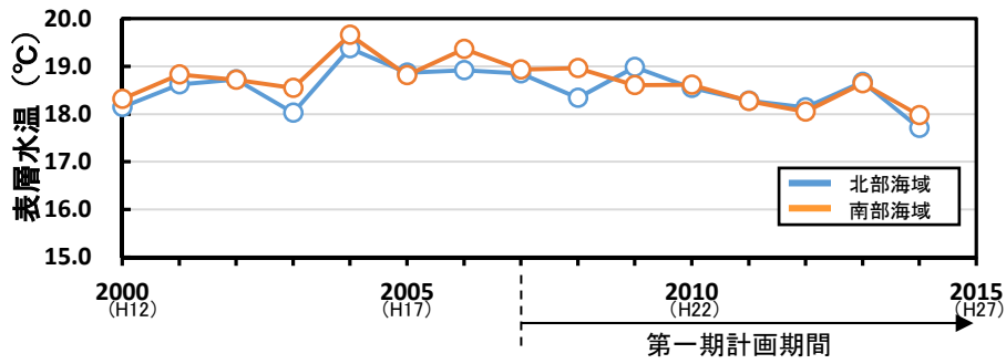
(1) 表層水温
