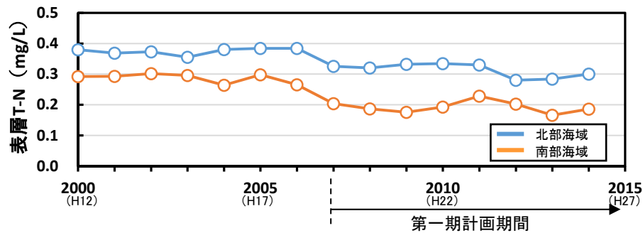
(3) 表層 T-N
