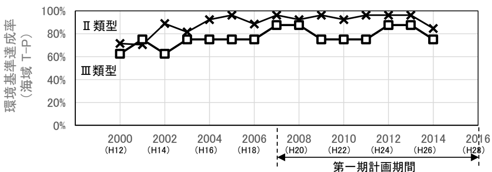
(3) T-P(海域)
