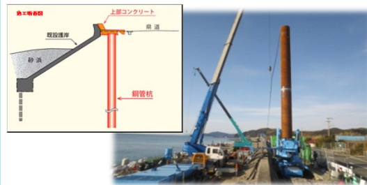
▲海岸堤防の補強（事例）
