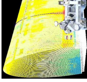
高精度MMSレーザを用いたコンクリート構造物3次元計測技術
