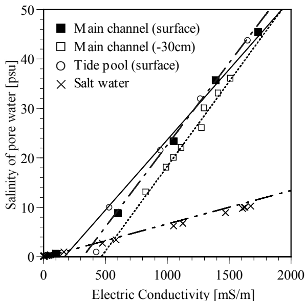
図-5 河床材料の電気伝導度と間隙水塩分濃度の関係
