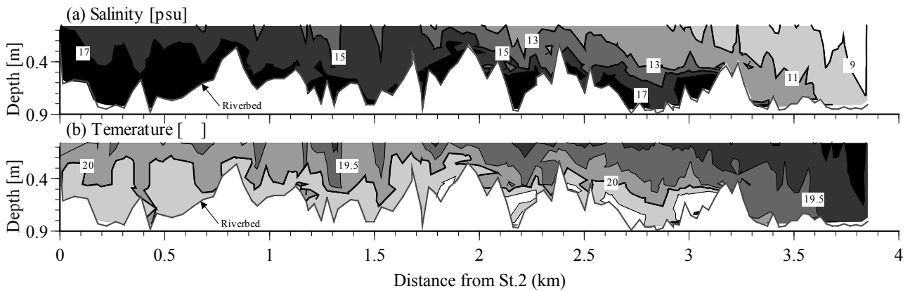
図-2 太田川放水路 St.2～3 における塩分・水温プロファイル（2005年5月22日，上段：塩分，下段：水温）。
