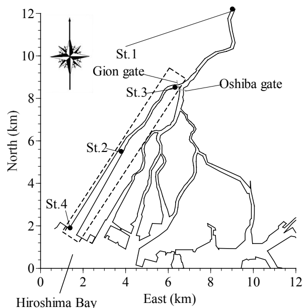
図-1 太田川感潮域の調査地点（破線枠は放水路）。
