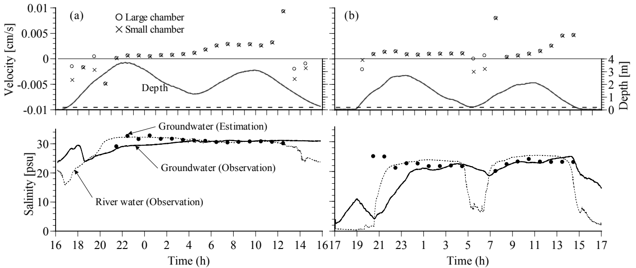
図-7 測定地点の水深と河床面を通じた推定流出速度(上段),河床地盤中の間隙水塩分濃度の実測値と推定値,および河川水の塩分濃度(下段)。(a)St. 2, (b)St. 3)。上図の破線はチャンバーが干出する水深を示す。
