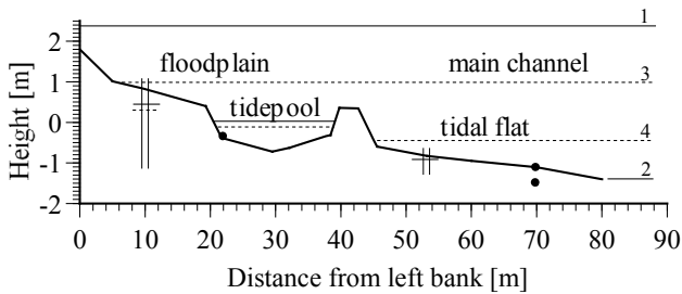
図-3 St.2 における河道横断形状 . 1, 2 : 大潮期の満潮位と干潮位 , 3, 4 : 小潮期の満潮位と干潮位 . 縦 2 重線 : 観測井戸 , : 試料採取位置 .
