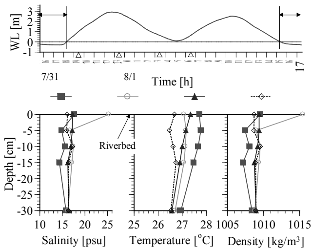
図-8 St.2における河床面を基準とした水位および低水路河床面以下での塩分・水温・密度プロファイル。図中の矢印は河床面の干出期間を示している。
