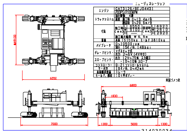
図-2 スリップフォームペーバの仕様概略図
