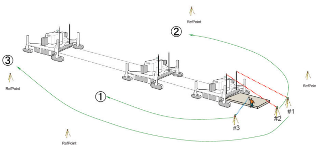
図-3 TSのターニング概念 (#1, 2, 3)
