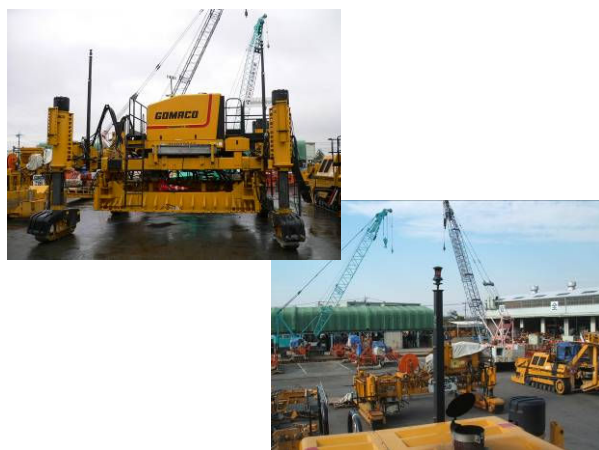
写真-6 360°プリズム (機械視準用×2台)
