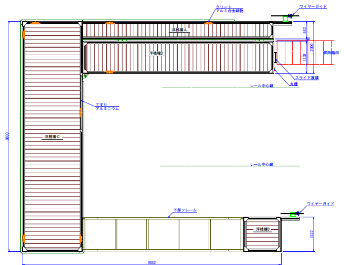
浮棧橋平面圖
