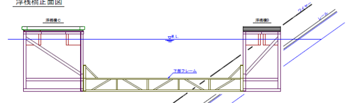
浮棧橋正面図
