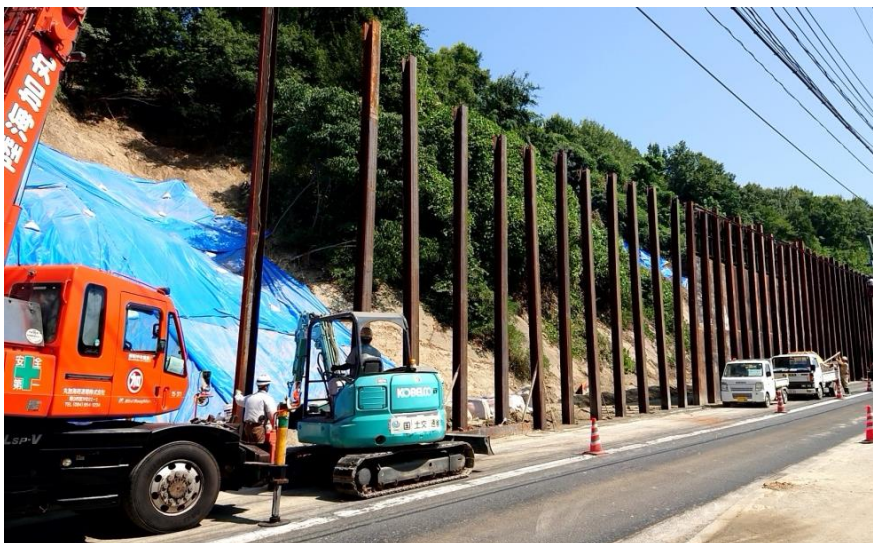
土工用防護柵設置支援（尾道市美ノ郷町）
