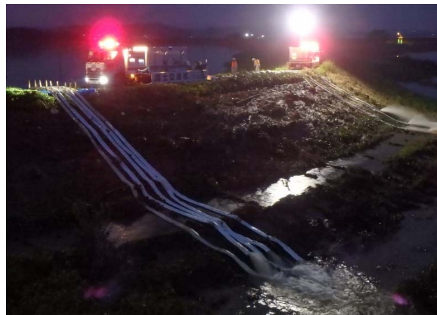
【宮城県・吉田川】排水ポンプ車による排水作業（応急対策班）
