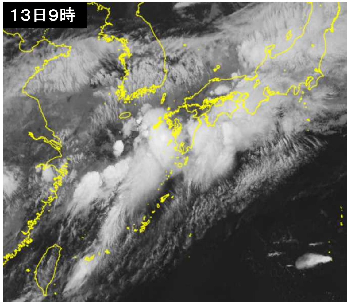
気象衛星(赤外画像)
