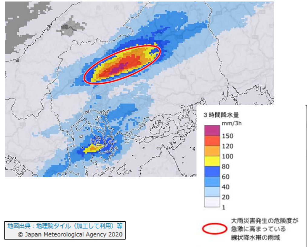
3時間降水量の様子
