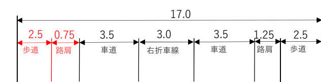
計画断面図 (単位: m)
