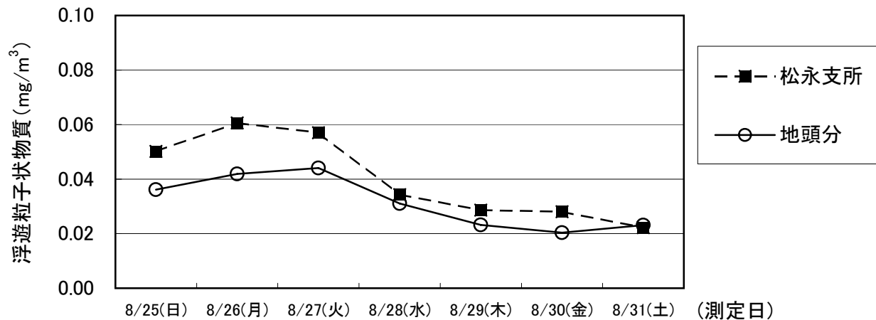
夏季:大気質調査結果(浮遊粒子状物質:SPM～日平均値～)
