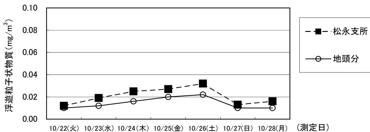
秋季:大気質調査結果(浮遊粒子状物質:SPM～日平均値～)
