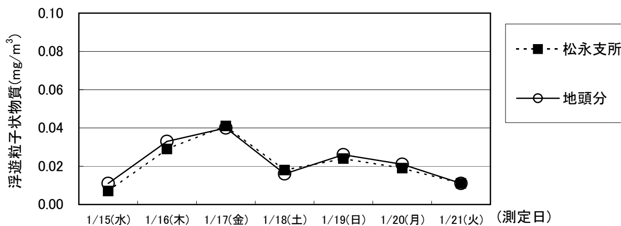
冬季:大気質調査結果(浮遊粒子状物質:SPM~日平均値~)
