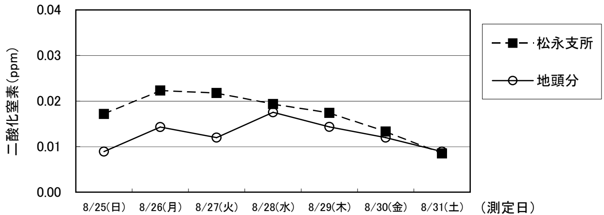
夏季:大気質調査結果(二酸化窒素:NO 2 )
