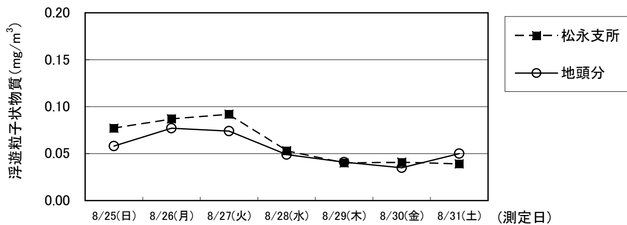
夏季:大気質調査結果(浮遊粒子状物質:SPM～時間最大値～)
