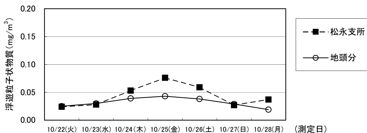
秋季:大気質調査結果(浮遊粒子状物質:SPM～時間最大値～)
