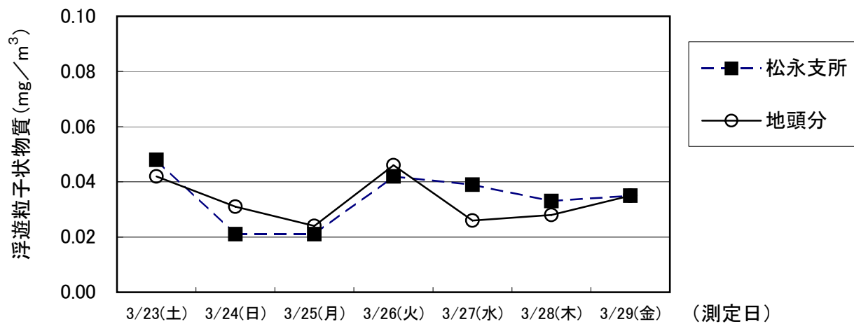
春季:大気質調査結果(浮遊粒子状物質:SPM～日平均値～)
