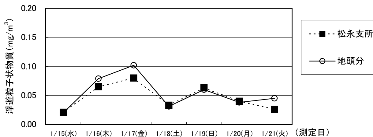
冬季:大気質調査結果(浮遊粒子状物質:SPM~時間最大值~)
