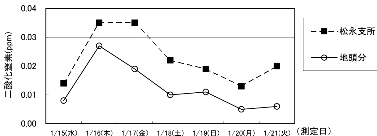
冬季:大気質調査結果(二酸化窒素:NO 2 )
