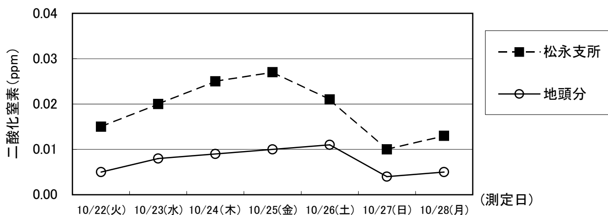
秋季:大気質調査結果(二酸化窒素: \text{NO}_2 )
