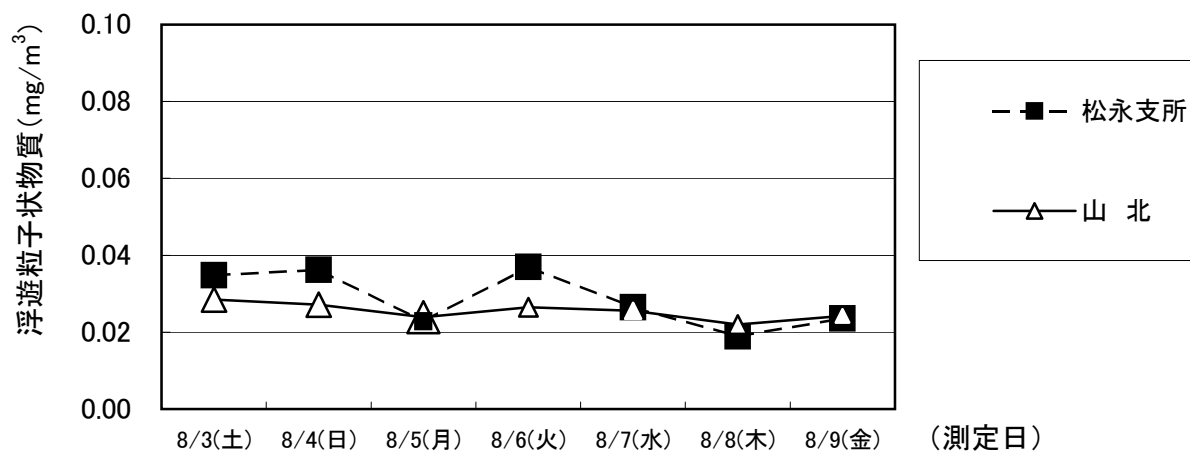
夏季:大気質調査結果(浮遊粒子状物質:SPM～日平均値～)
