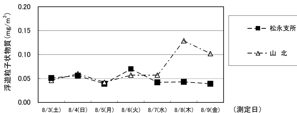
夏季:大気質調査結果(浮遊粒子状物質:SPM～時間最大値～)
