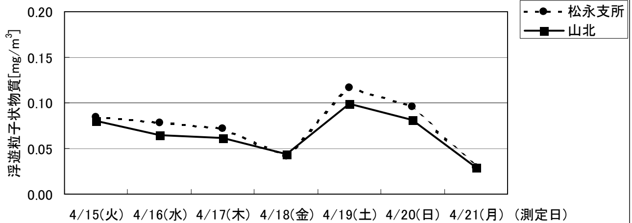
春季:大気質調査結果(浮遊粒子状物質:SPM～時間最大値～)
