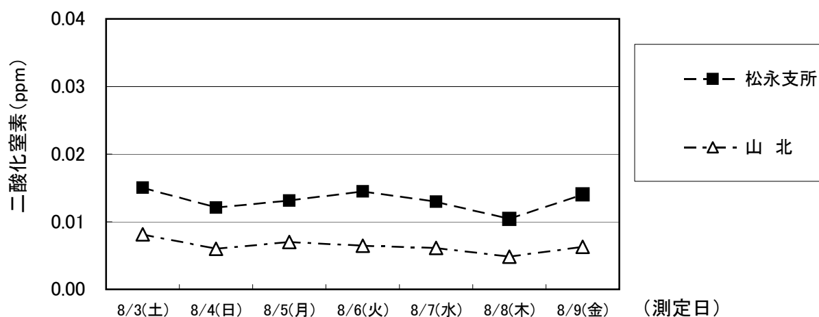
夏季:大気質調査結果(二酸化窒素:NO 2 )
