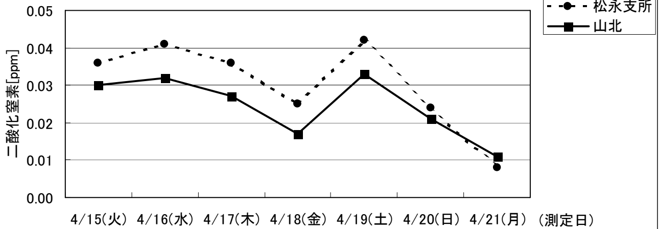
春季:大気質調査結果(二酸化窒素:NO 2 )
