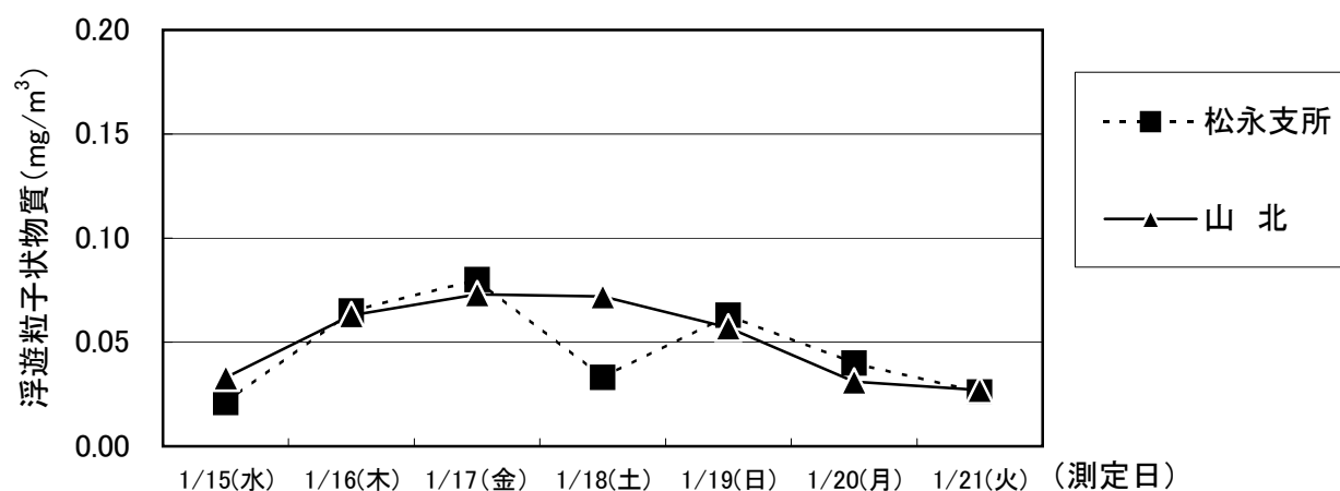
冬季:大気質調査結果(浮遊粒子状物質:SPM～時間最大値～)
