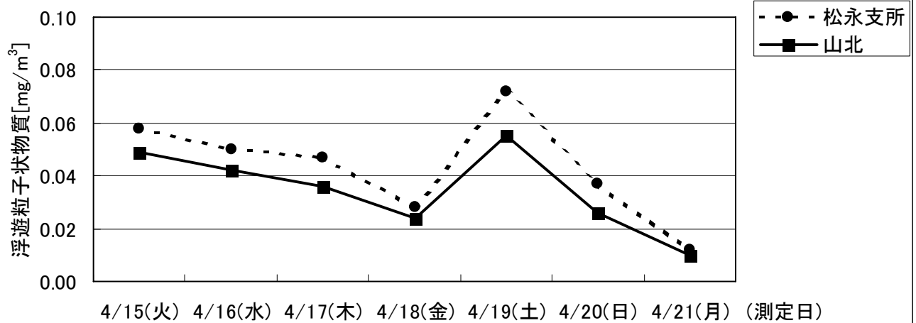
春季:大気質調査結果(浮遊粒子状物質:SPM～日平均值～)
