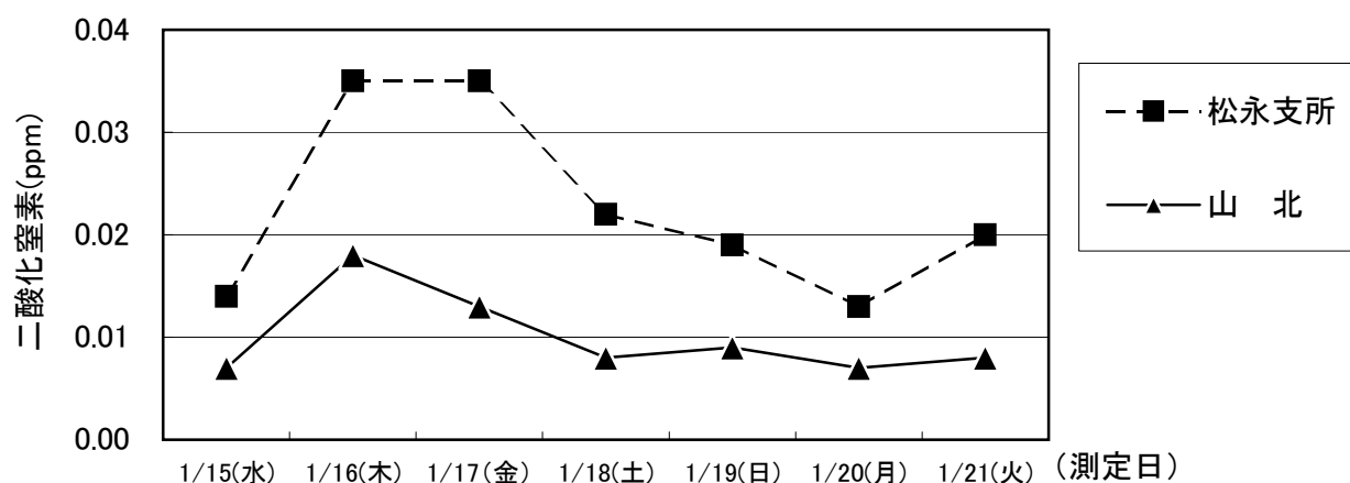
冬季:大気質調査結果(二酸化窒素:NO 2 )
