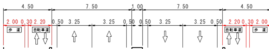
【計画断面図 (案)】
