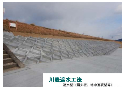
堤防浸透対策工法 （川表遮水工法）
