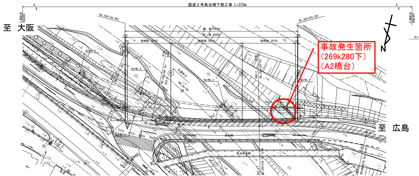
平面図 S=1:300
