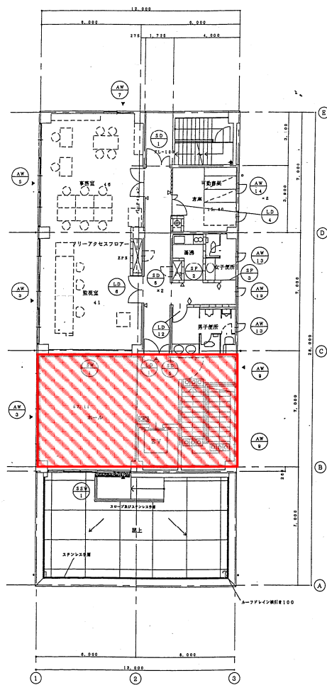
3階平面図
