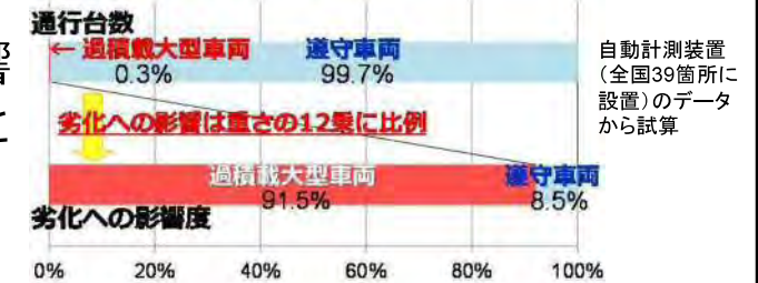
【図 道路橋の劣化に与える影響】
