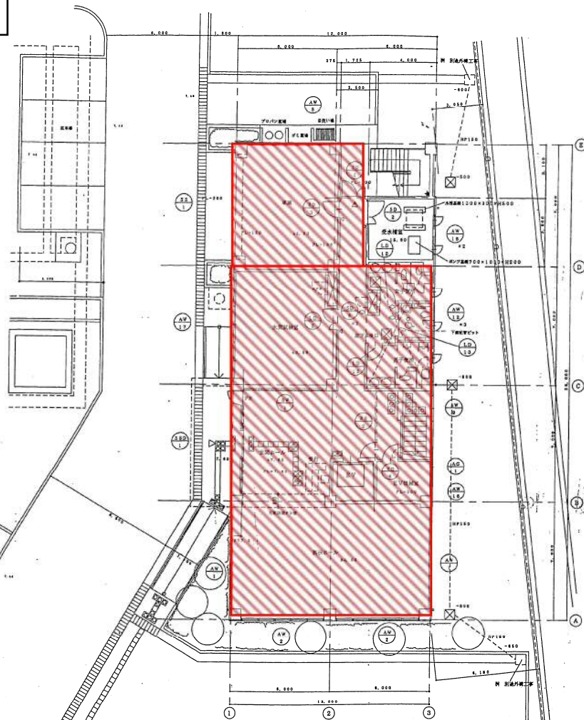
1階平面図
