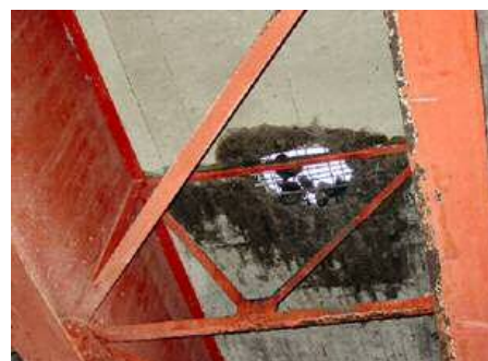
橋の裏面の様子(床版)
