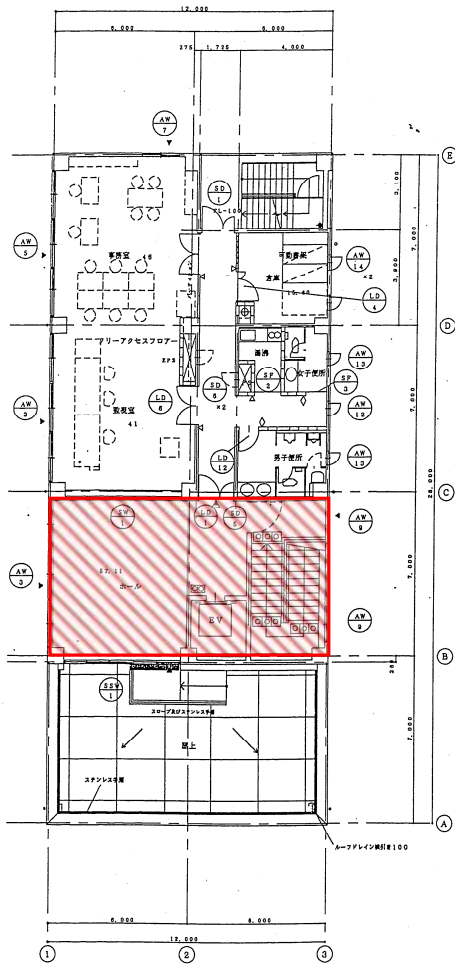
3階平面図
