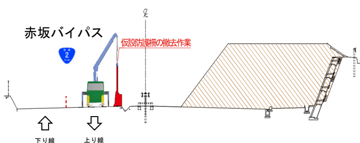
仮設防護柵撤去状況
