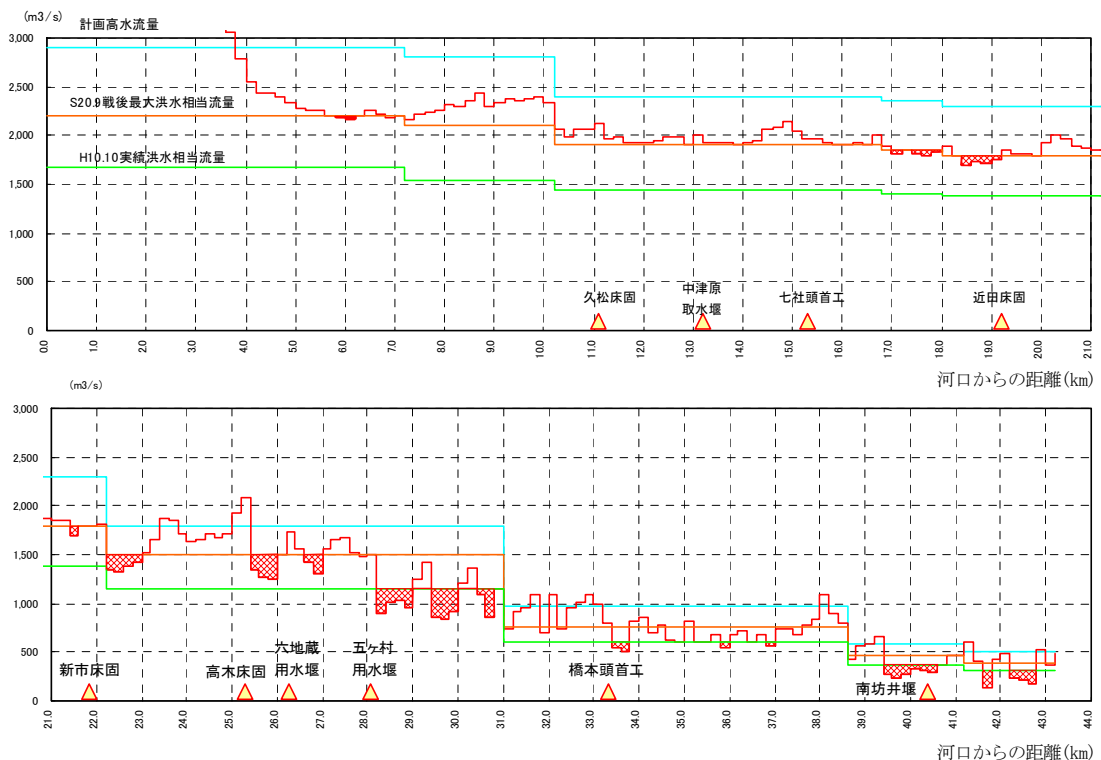
図 2-1-1 流下能力図
