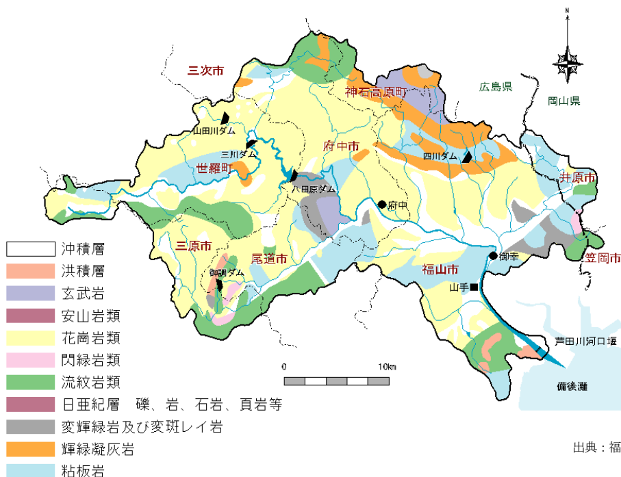
図 1-1-3 地質図
