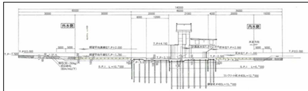
断面図
