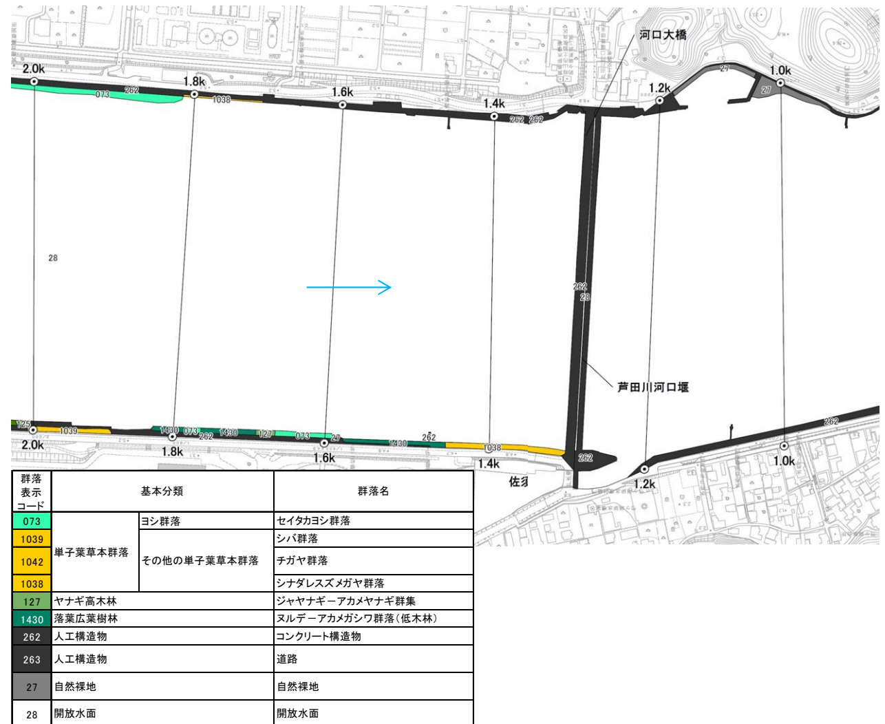
【芦田川河口堰付近の植生図（平成30年度）】
