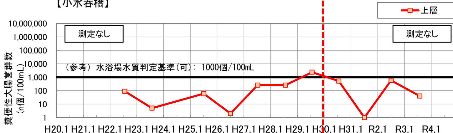
【小水呑橋】
