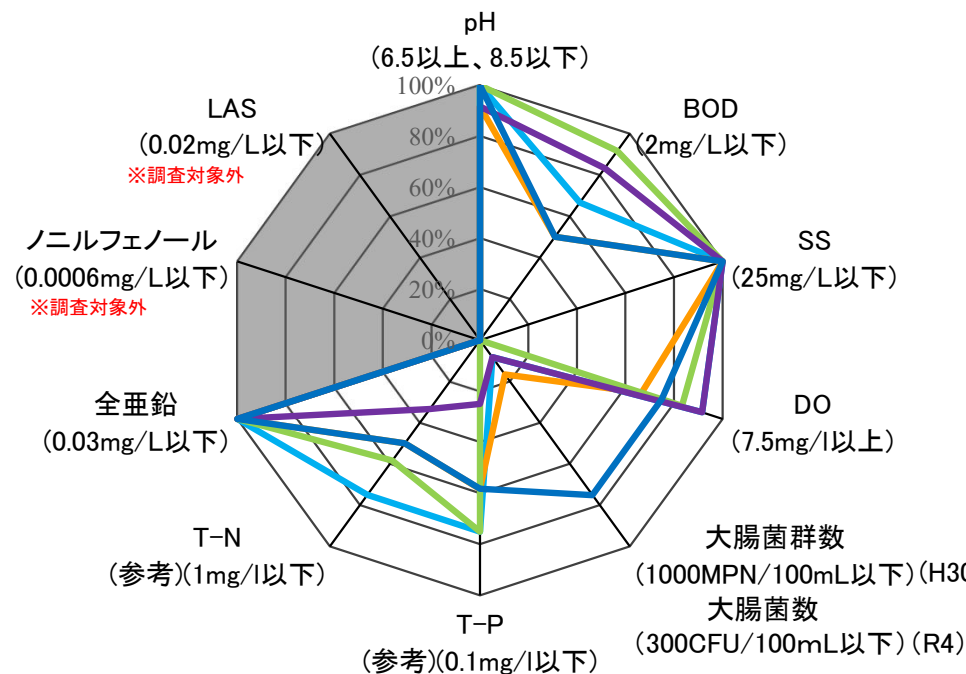
【本川山手】
