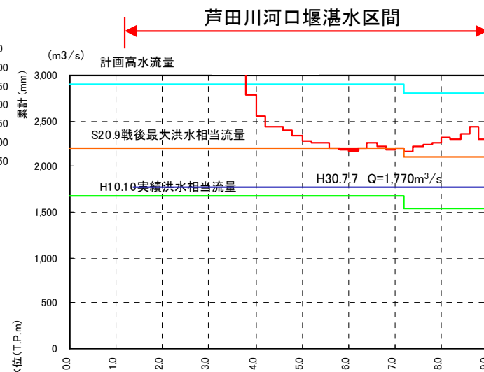
芦田川の流下能力図 (芦田川水系河川整備計画【国管理区間】 H20.2)
