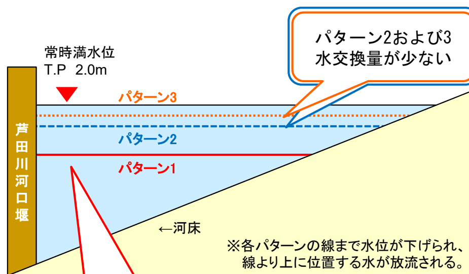
【弾力的放流時の水交換イメージ】
