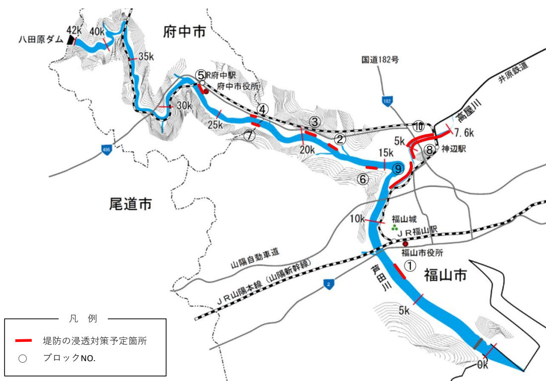
29 図 5-1-10 堤防の浸透対策の実施箇所
