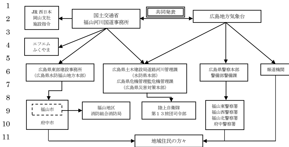
図 5-2-4 洪水予報の伝達経路
