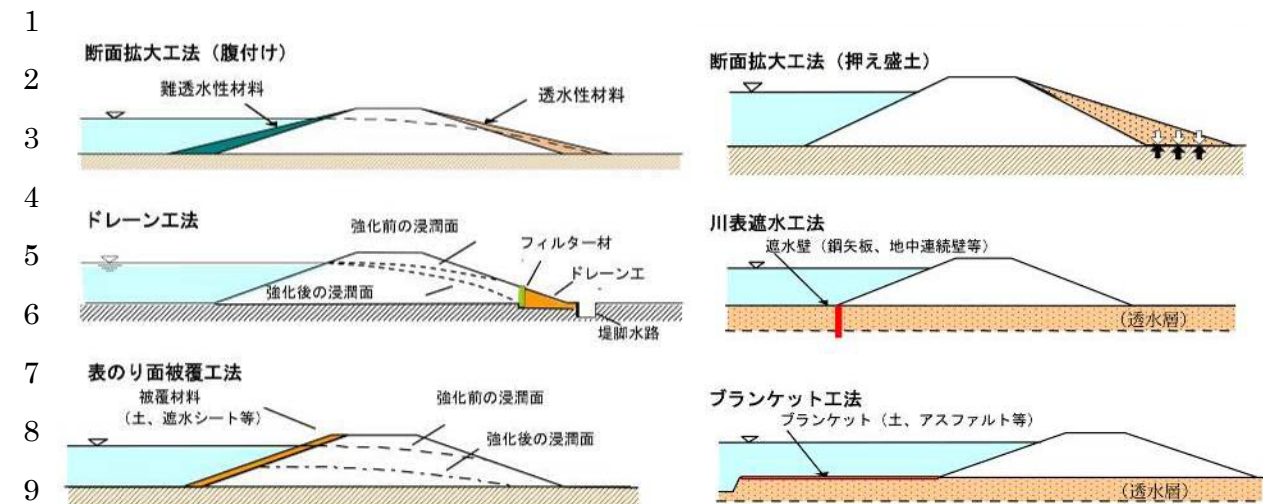
図 5-1-11 堤防浸透対策工法イメージ図（各種対策工法）
