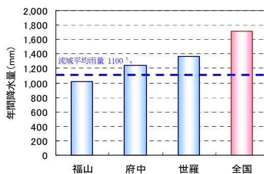
※気象庁観測所のデータに基づき作成 全国は昭和 46 年～平成 12 年の平均値 その他の観測所は平成 9 年～平成 18 年の平均値 図 1-1-5 気象庁観測地点の年間降水量の比較
