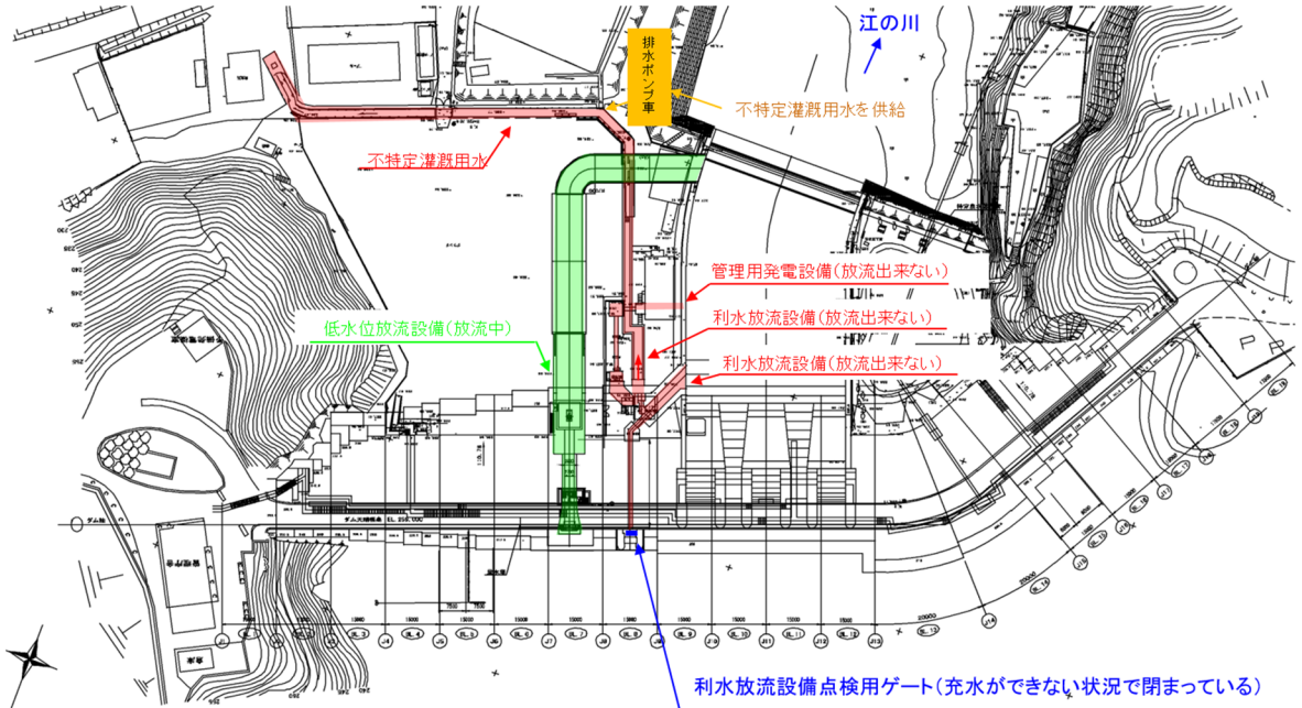
ダム平面図
