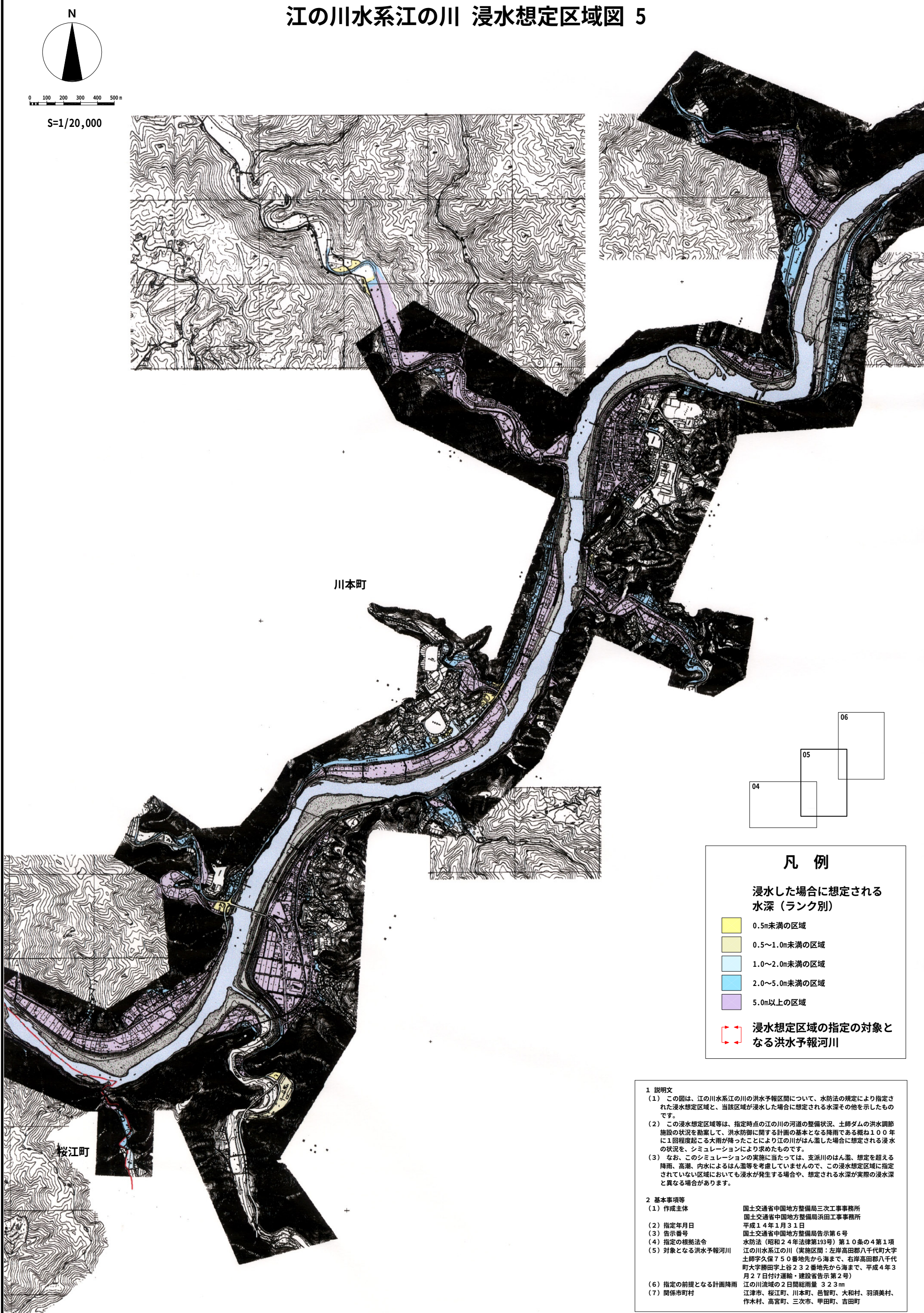
図-4.2.6 江の川水系江の川 浸水想定区域図 5
