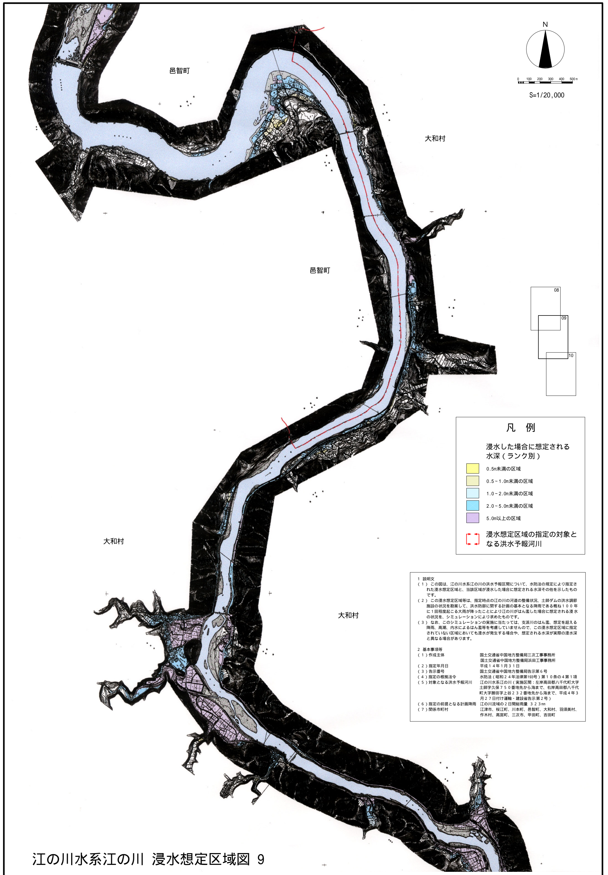
図-4.2.10 江の川水系江の川 浸水想定区域図 9
