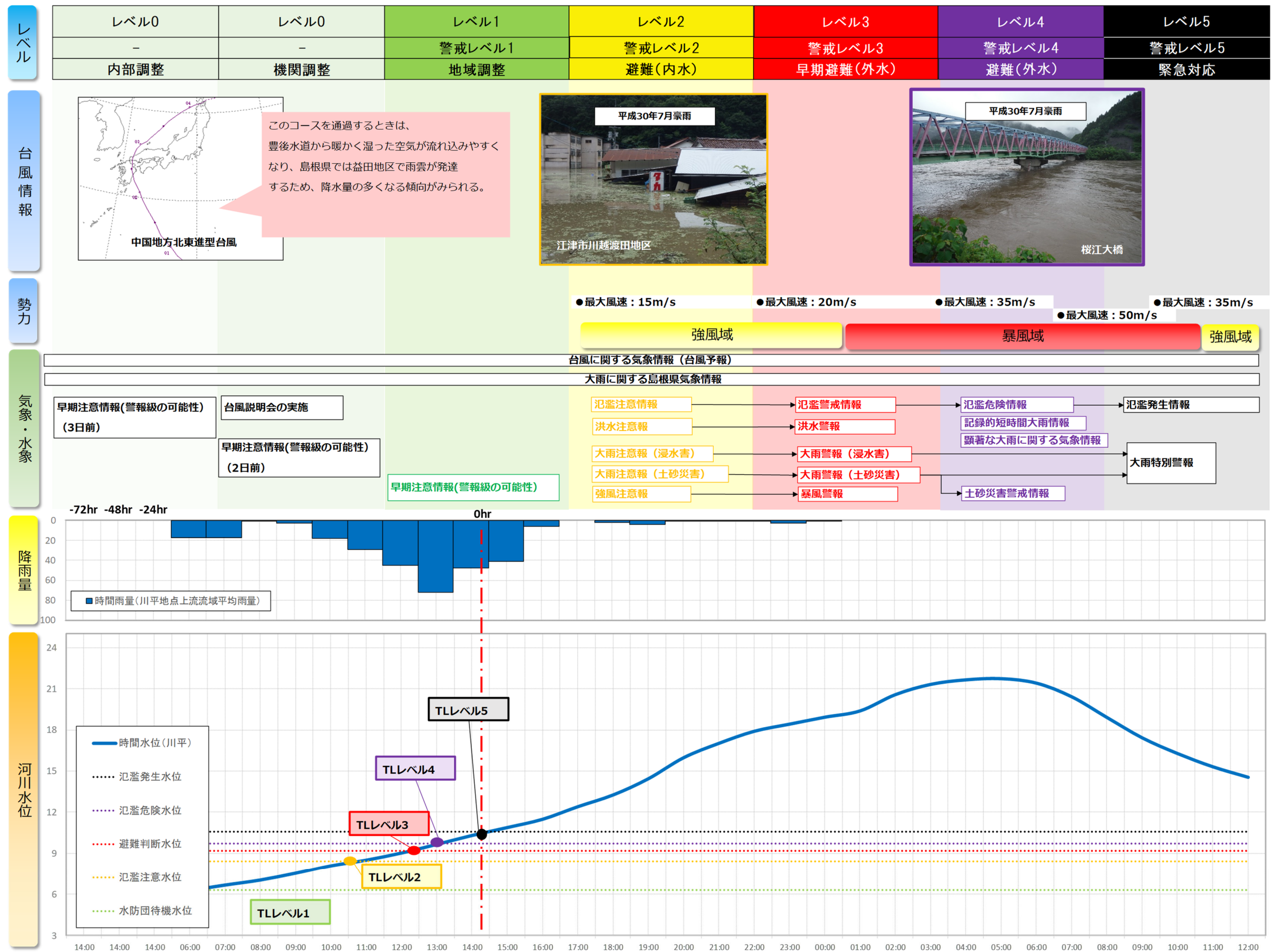
図 5 江の川(下流)水害タイムライン令和6年度版 想定シナリオ
