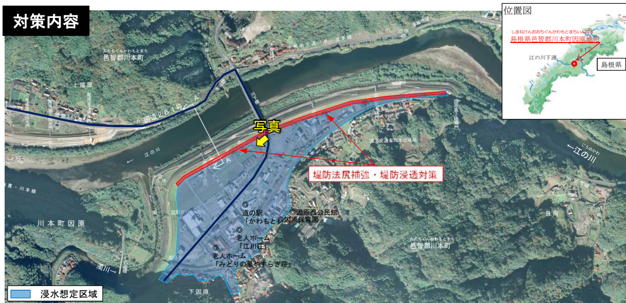
施工イメージ（A-A'）
