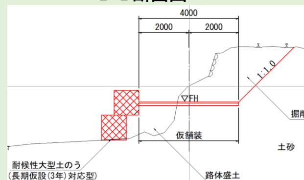
B-B断面図
