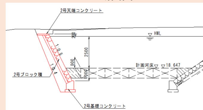
A-A断面図
