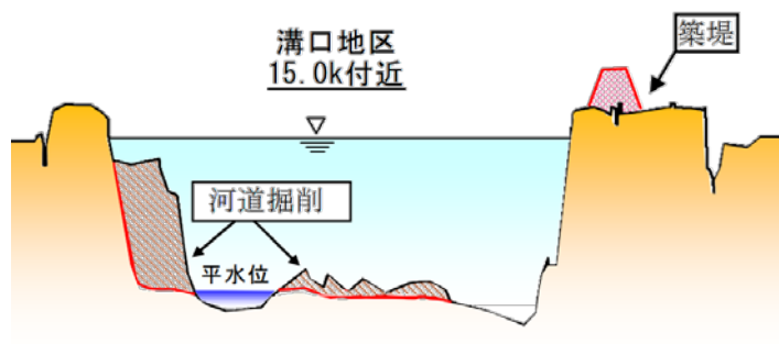
河道掘削・築堤のイメージ図
