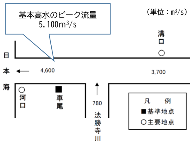
河川整備基本方針の流量配分図
