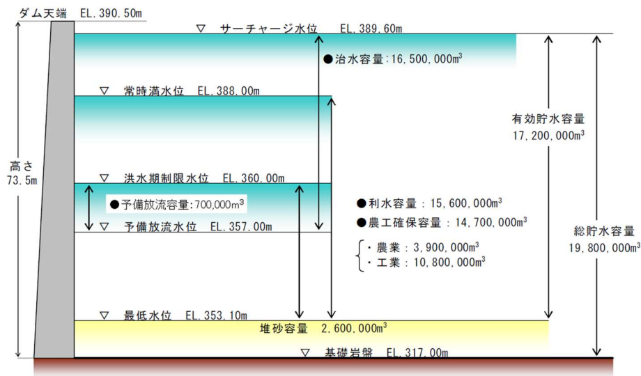
菅沢ダム 貯水池容量配分図
