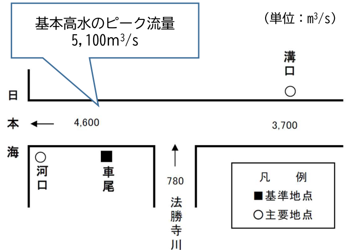
河川整備基本方針の流量配分図
