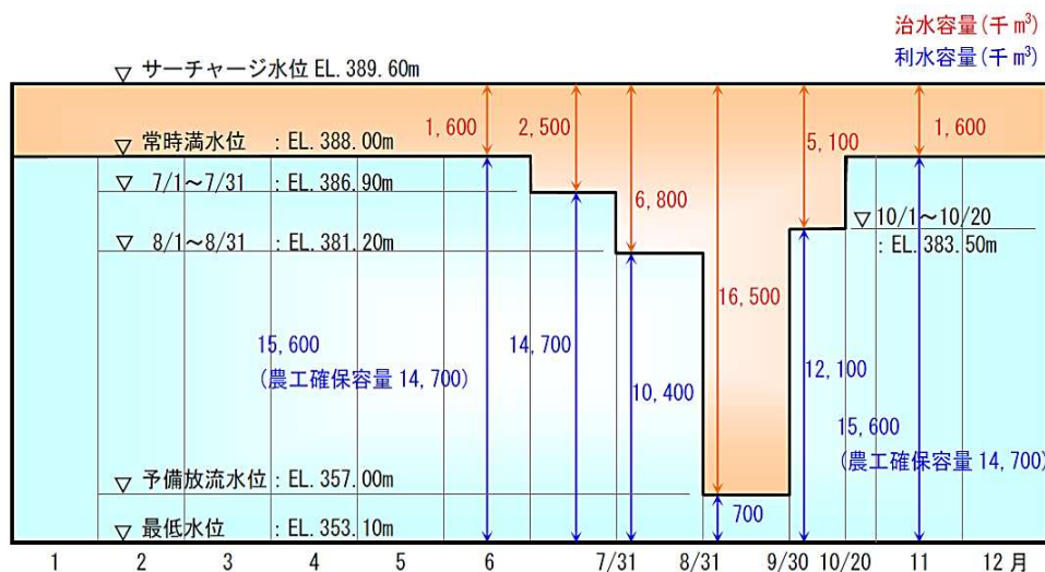
菅沢ダム 期別貯水池運用パターン
