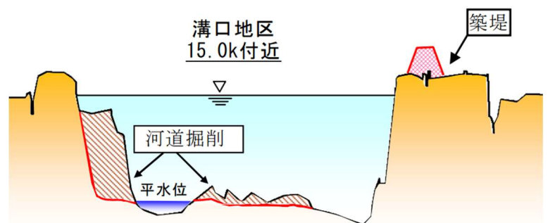
河道掘削・築堤のイメージ図
