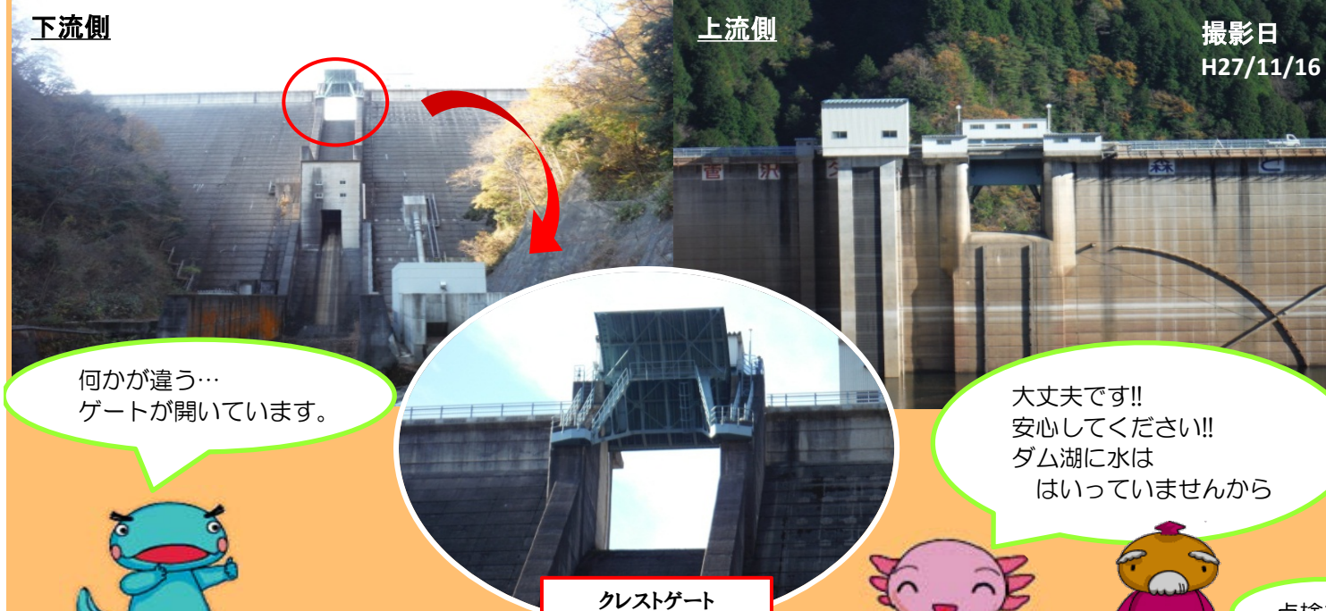
クレストゲート (非常用洪水吐設備)
