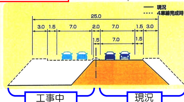
四車線化断面図
