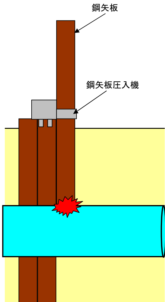
鋼矢板圧入側面図
