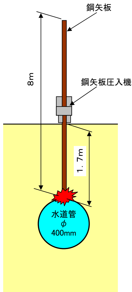
鋼矢板圧入正面図
