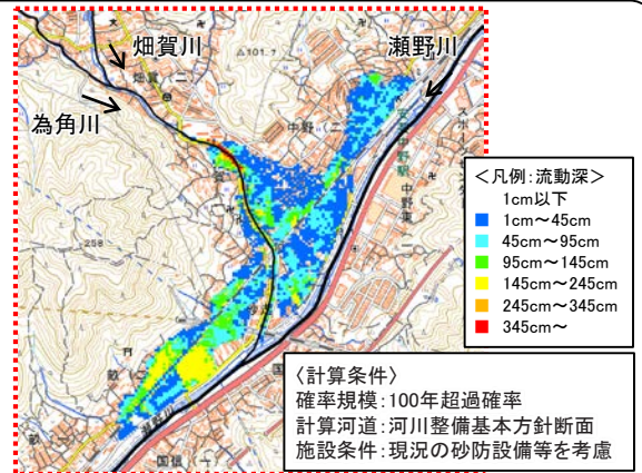
畑賀川合流点付近の土砂・洪水氾濫の想定範囲
