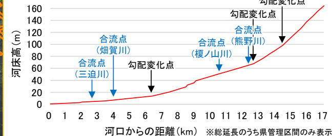
瀬野川本川の縦断面図
