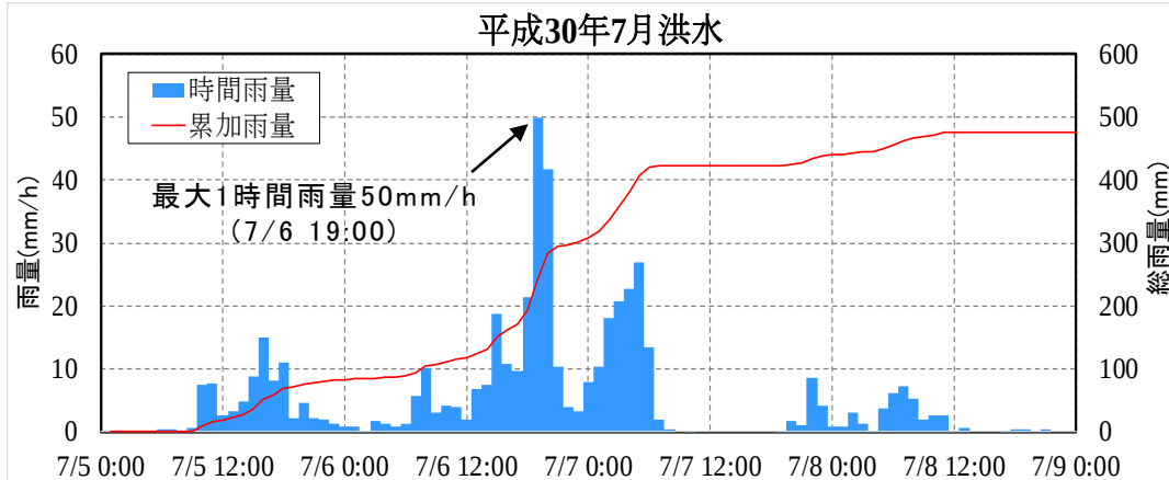
平成30年7月5日～9日の降雨(瀬野川流域平均雨量)
