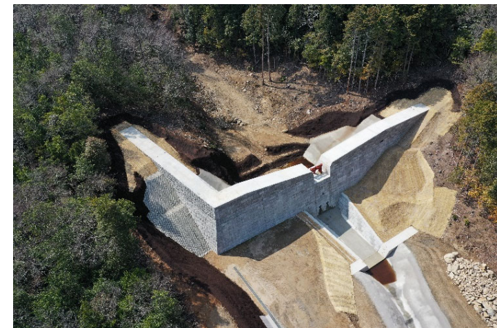
砂防堰堤施工状況③
