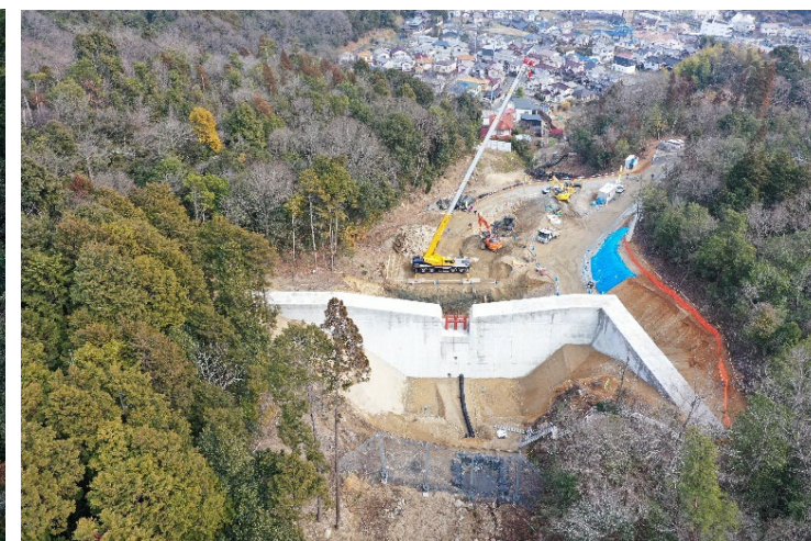
砂防堰堤施工状況③
