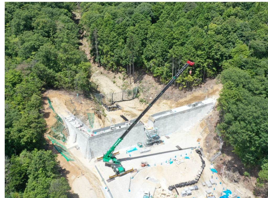
砂防堰堤施工状況②
