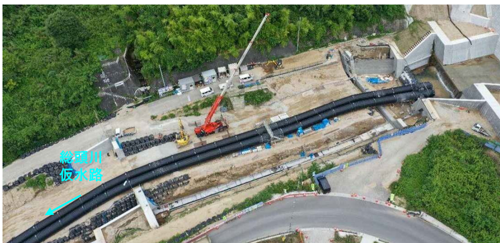
【総頭川遊砂地】
