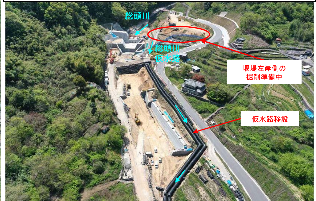
【施工状況（下流から上流を望む）（R6. 4月中旬時点）】
