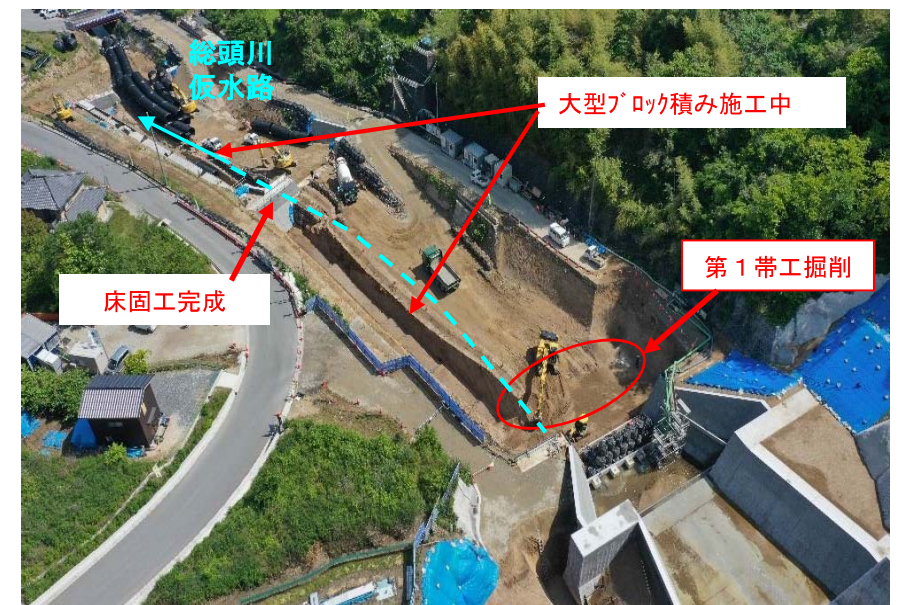
【大型ブロック積施工状況(上流から下流を望む)】
