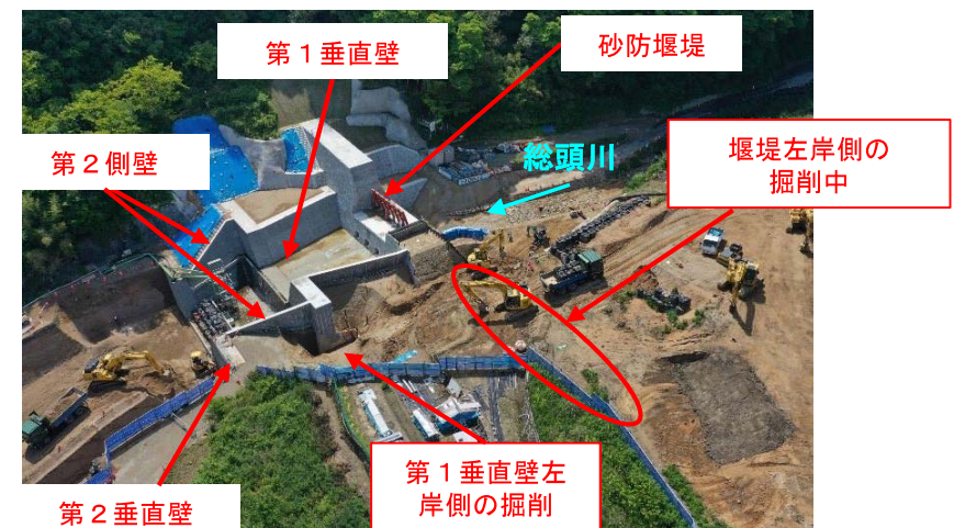
【砂防堰堤の施工状況（上空から望む）】
