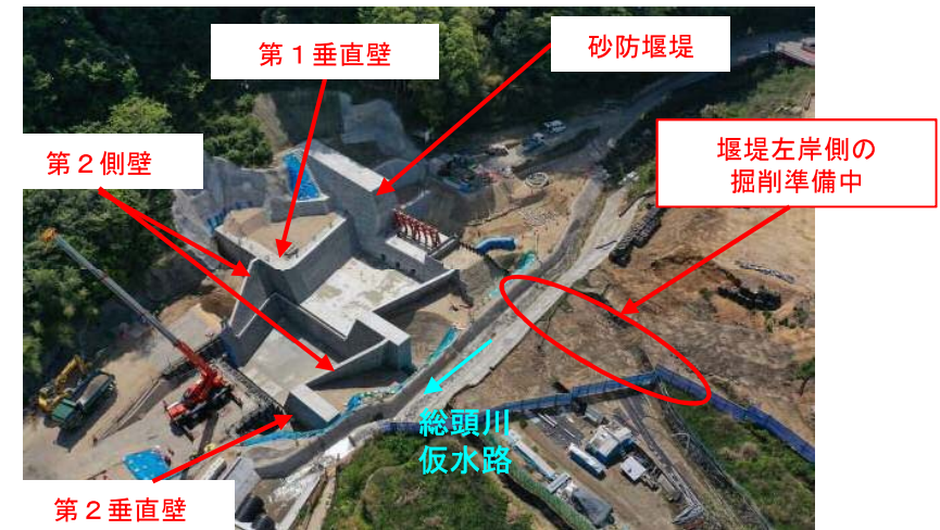
【砂防堰堤及び垂直壁の状況（上空から望む）】
