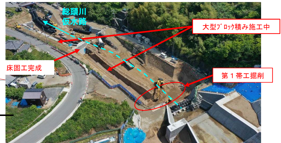
【大型ブロック積み施工状況（上流から下流を望む）】
