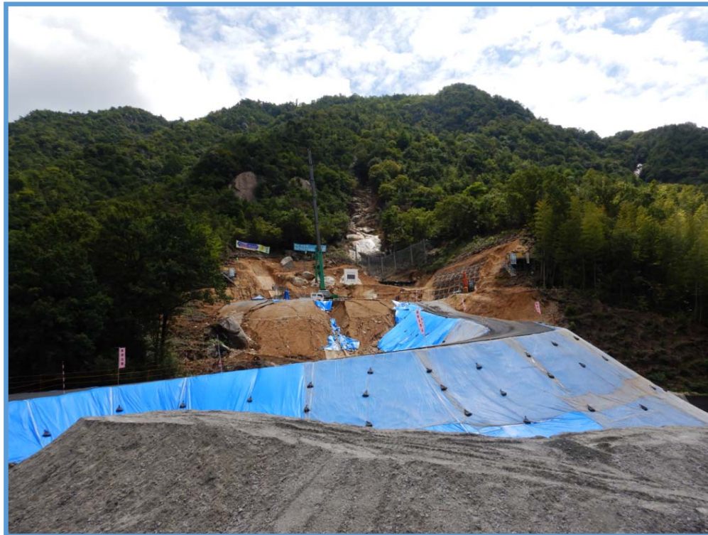
砂防堰堤の本体掘削状況 ①
