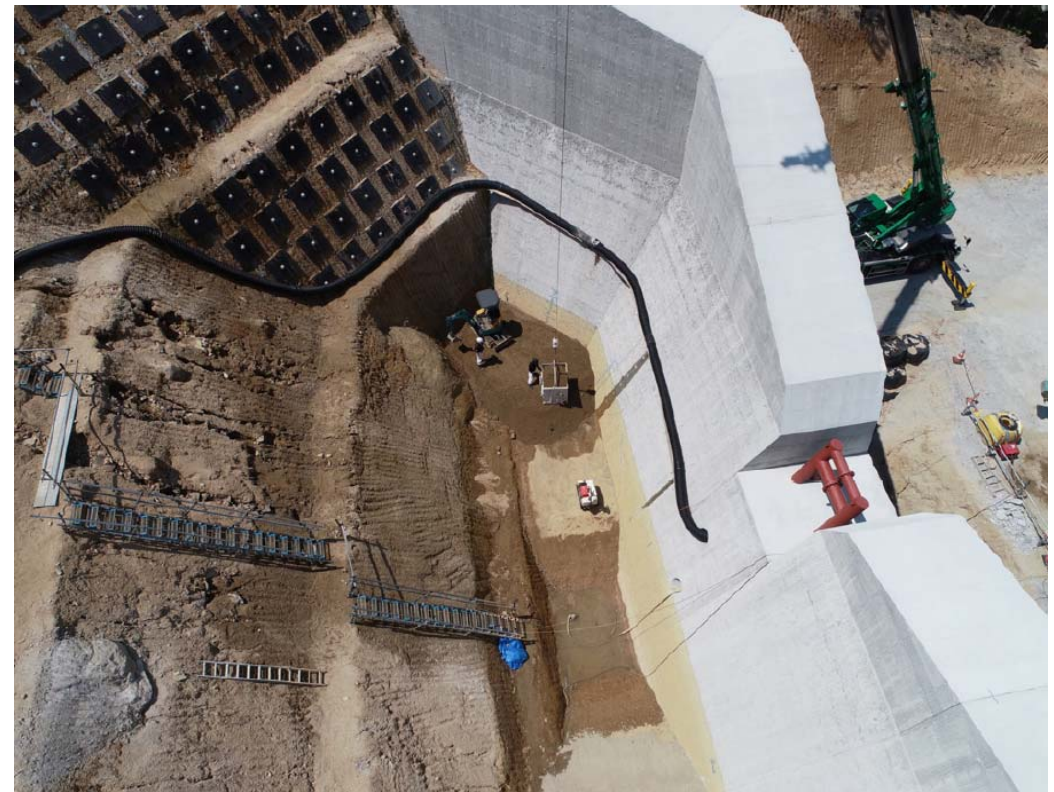
砂防堰堤の埋戻し施工状況
