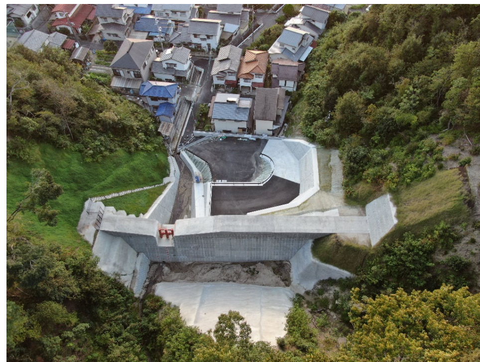
砂防堰堤全景（上流側より）
