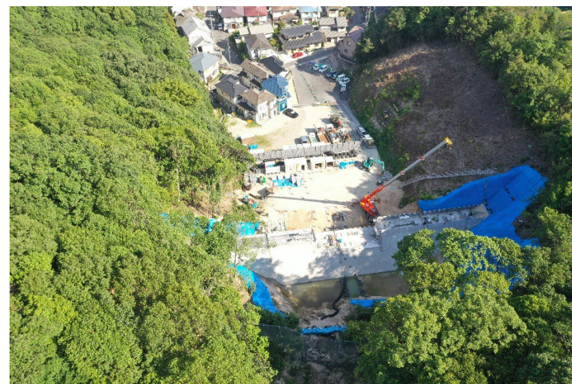
【施工状況（上流側より）】
