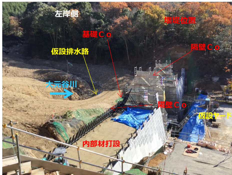
堰堤コンクリート施工①
